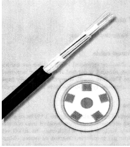
الشكل 3-20 مثال على تكنولوجيا ليف اللب المثقوب، غير المعدني (تقدمة شركة كورنينغ لأنظمة الأسلاك)
